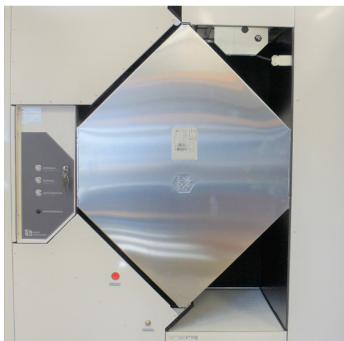
Motströmsvärmväxlare i aluminium med mer än 80% temperaturverkningsgrad.
