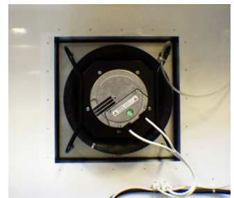
Frånluftfläkt insida
